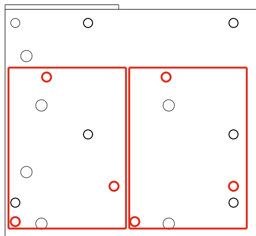
Расположение расширителей NV 2124
