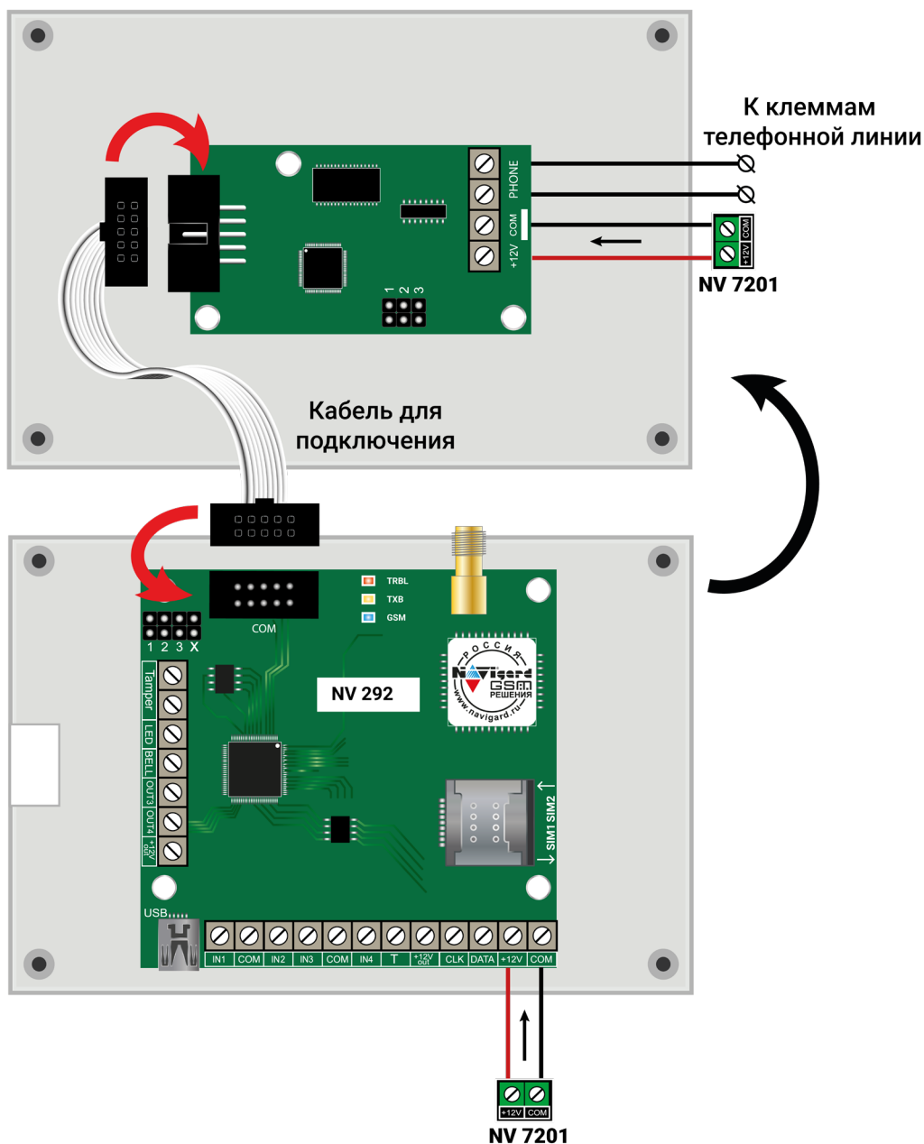
Рисунок 1. Подключение модуля согласования
